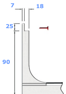
Doorsnede tegellip
